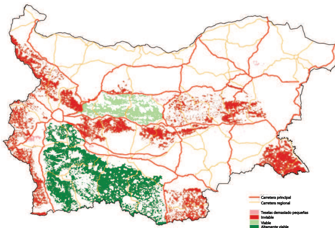
Figura 4.6.1. Viabilidad de la población de osos antes de aplicar medidas de desfragmentación. Modelo LARCH aplicado en Bulgaria. Fuente: van der Grift et al. (2008).
