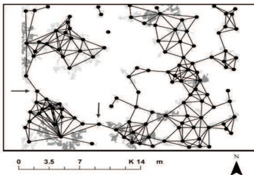
Figura 4.8. Paisaje representado en términos de la teoría de grafos. Los parches son áreas continuas de hábitat potencial de zorzal manchado ( Hylocichla mustelina ). Los nodos (círculos negros) están representados en el centro de los parches. Se muestran los enlaces entre nodos separados como máximo 2,5 km. Las flechas indican nodos críticos para el mantenimiento de la conectividad del conjunto. Fuente: Urban (2005).
