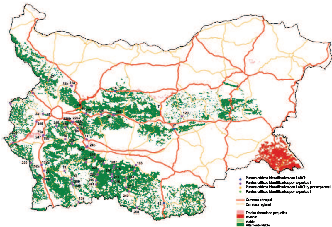
Figura 4.6.2. Viabilidad de la población de osos antes después de aplicar medidas de desfragmentación. Modelo LARCH aplicado en Bulgaria. Fuente: van der Grift et al. (2008).
