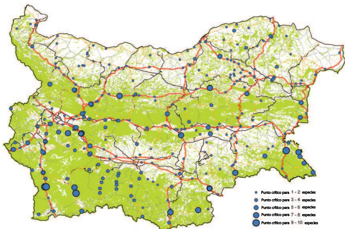
Figura 4.7. Puntos críticos para la conectividad identificados en Bulgaria. Modelo LARCH. Fuente: van der Grift et al. (2008).
