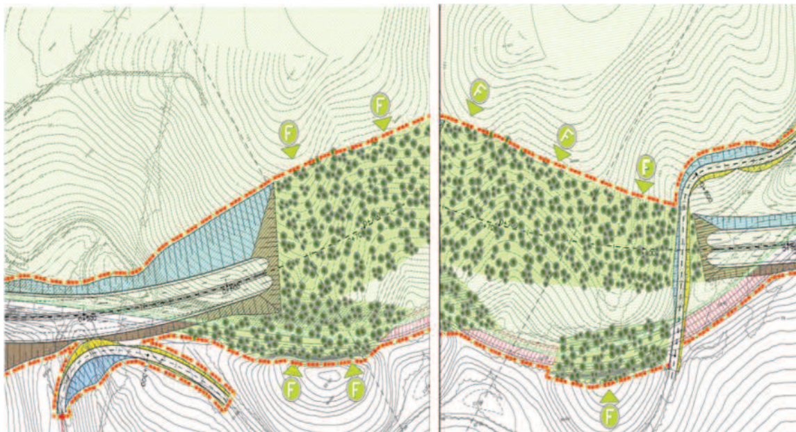
Figura 6.13. Propuesta de ecoducto incorporado en el estudio de impacto ambiental del desdoblamiento de la carretera C-66 en el tramo Palafrugell-Forallac. Fuente: GISA, 2006a.
