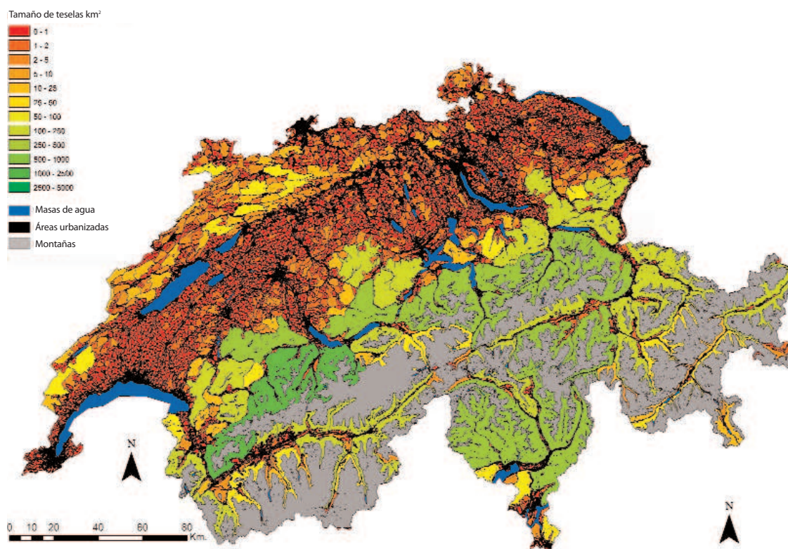
Figura 4.2. Fragmentación del paisaje en Suiza en el año 2002 evaluada a partir de la aplicación del método de tamaño efectivo de malla. Fuente: Jaeger et al. (2010).
