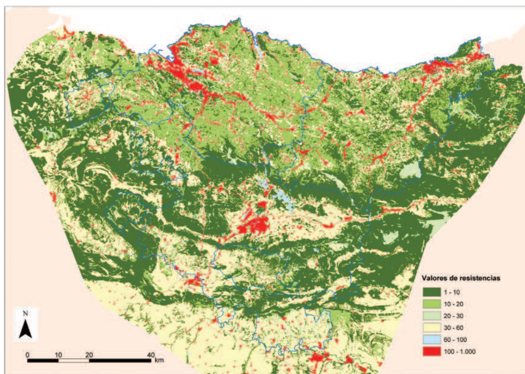
Figura 6.1. Mapa de resistencias de los usos del suelo al desplazamiento de las especies objetivo de la red de Corredores Ecológicos del País Vasco. Fuente: Gurrutxaga (2005).
