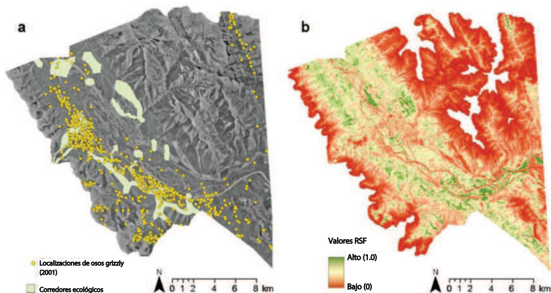
Figura 4.9. Aplicación de una función de selección de recursos RSF para evaluar o diseñar corredores de fauna. (a) Localizaciones por radioseguimiento de tres osos grizzli en la región de Canmore (Alberta, Canadá) durante el año 2001; en verde, los corredores de fauna declarados. (b) Se desarrolló una función de selección de recursos mediante regresión logística comparando las variables topográficas y de vegetación en los puntos donde se localizaron osos y en puntos al azar dentro de las áreas de campeo combinadas de los tres osos. El mapa resultante (b) identifica las áreas con mayor probabilidad relativa de ocurrencia de osos (verde) y puede utilizarse para evaluar o modificar corredores existentes o para optimizar propuestas de nuevos corredores. Fuente: Chetkiewicz et al. (2006).
