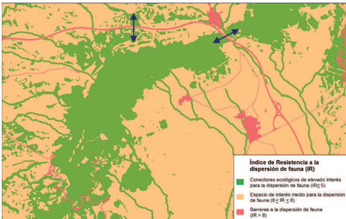
Figura 4.5. Cartografía elaborada mediante el modelo DISPERSA basado en el análisis de resistencia de los usos del suelo al desplazamiento de las especies objetivo. Las flechas indican posibles zonas a desfragmentar en puntos de cruce de una carretera con sectores de alto interés para la conectividad. Fuente: Modificado a partir de Minuartia.
