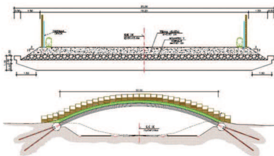
Figura 6.25. Secciones longitudinal y transversal de un paso superior. Fuente: Proyecto de Construcción: Pasos de fauna en A-483 y A-494. Junta de Andalucía (2008).
